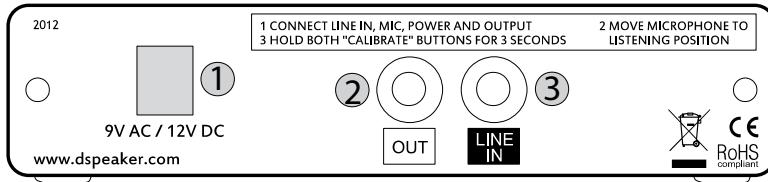
Abbildung 2: Anti-Mode 8033 cinema Rückansicht
