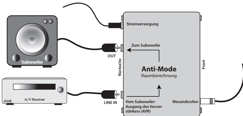
Abbildung 4: Anti-Mode 8033 anschliessen
