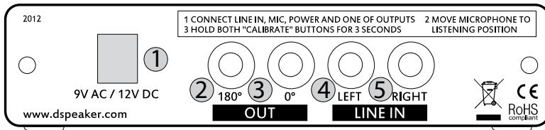
Abbildung 3: Anti-Mode 8033s-II Rückansicht
