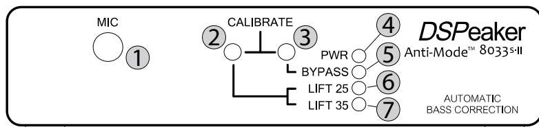
Abbildung 1: Anti-Mode 8033s-II Frontansicht
