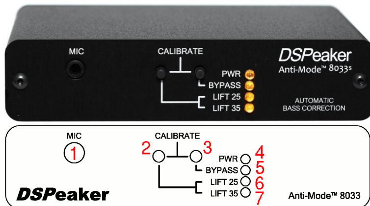
Kuva 1: ANTI-MODE 8033 etupaneeli
